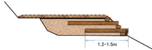
<횡 단면도>
