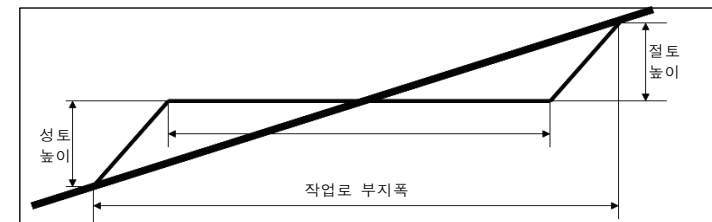
<작업로의 단면형태>
