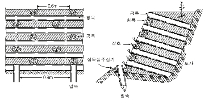
<정면도 예시>
